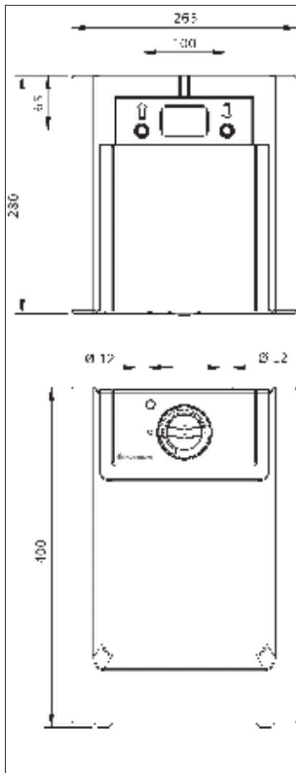
fig. 4 (Dimensions en mm)
