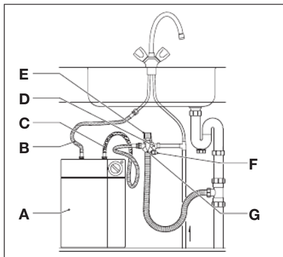
Fig. 2.1 Fonctionnement du système sous pression
