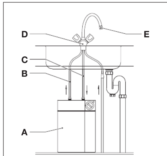
Fig. 2.2 Principewerking drukloos systeem
