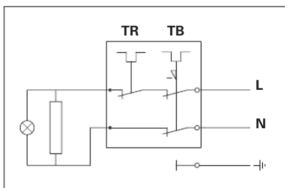
Fig. 2.3 Schéma de branchement électrique
