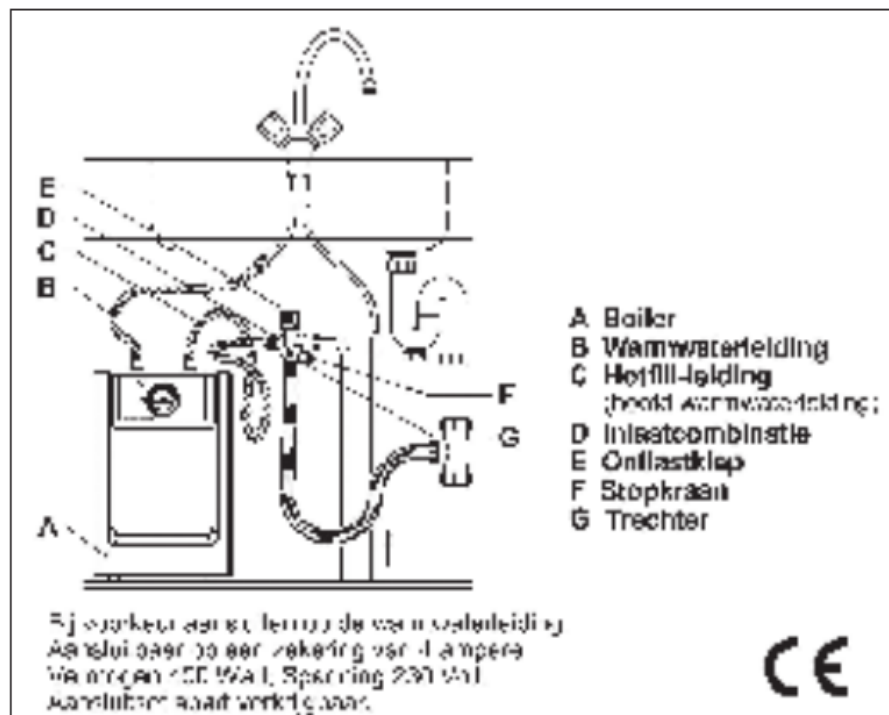
Fig. 5.2: Inventum Q10 Hotfill keukenboiler
