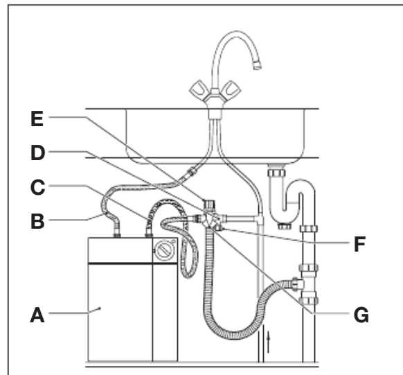
Fig. 2.1 Principewerking systeem onder druk
