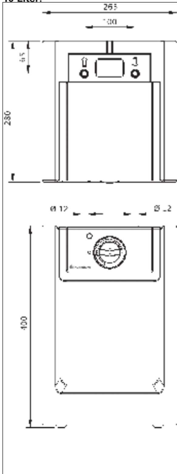
Fig. 4 (Afmetingen zijn weergegeven in mm)
