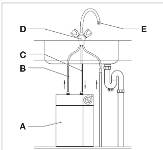
Fig. 2.2 Fonctionnement du système sans pression
